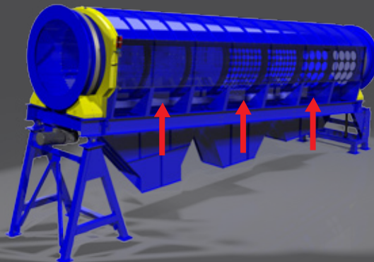
Le crible rotatif pour le traitement des particules fines
